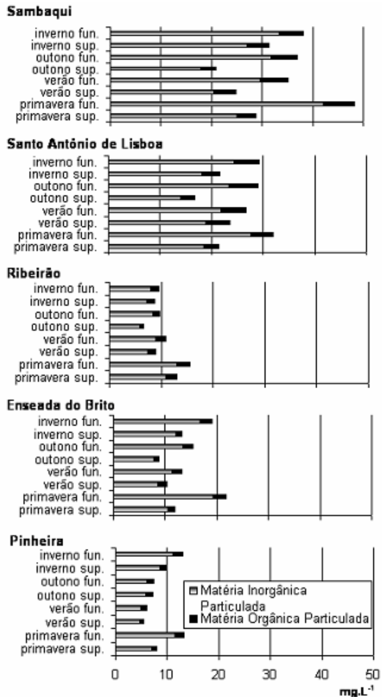
Figura 3. Quantidade e qualidade de MPT. MIP (mg.L -1 ) e MOP (mg.L -1 ) nos diferentes locais de amostragem. Dados de 1999 a 2002 agrupados em médias sazonais.
