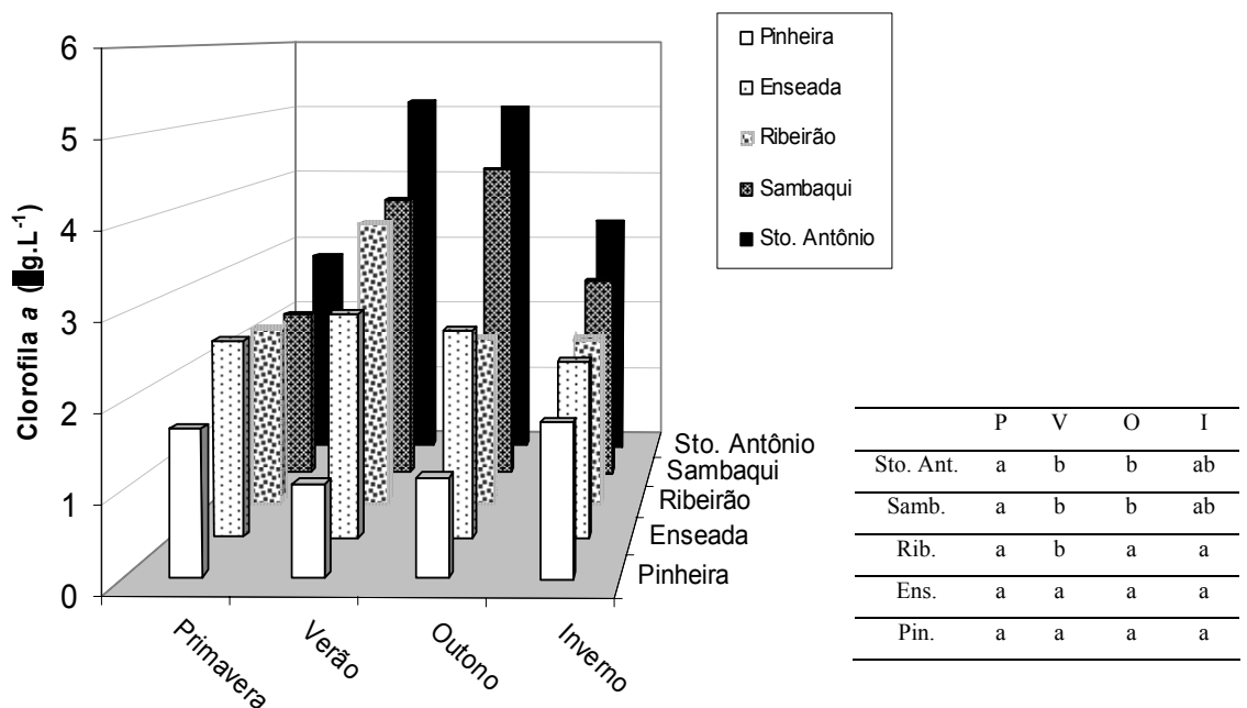
Figura 2. Variação sazonal da clorofila a ( \mu\text{g.L}^{-1} ) nos diferentes pontos de estuário, anos de superfície, de 1999 a 2002 médias sazonais de valores agrupados. Resultado de análise de Tukey entre as estações dentro de cada ponto.
